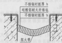
阻火带安装示意图
