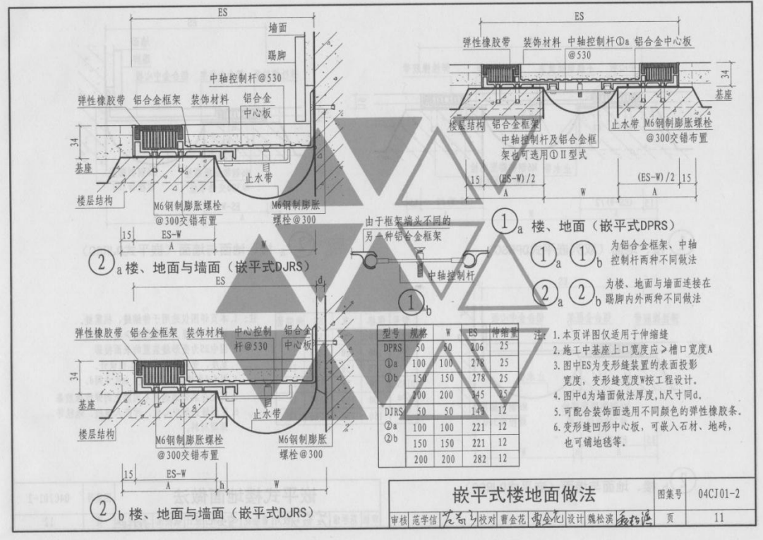
嵌平式楼地面做法 图集号 04CJ01-2 审核 范学信 范学信 校对 曹金花 曹金花 设计 魏松滨 魏松滨 页 10
