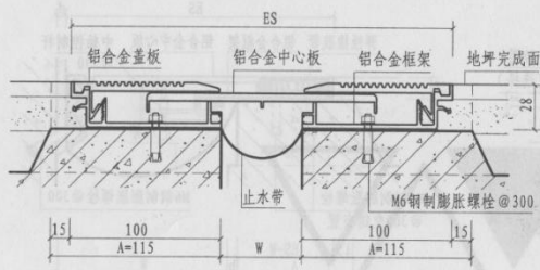
① 楼、地面 (卡锁式DPK)
