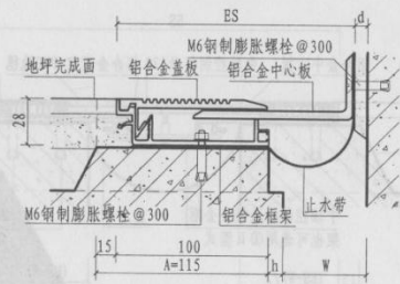
② 楼、地面与墙面 (卡锁式DJK)
