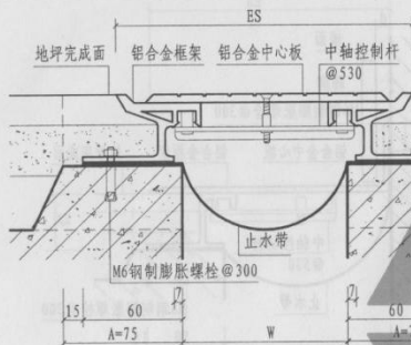
① 楼、地面 (防滑型DPF)
