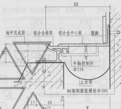
② a 楼、地面与墙面 (防滑型DJF)
