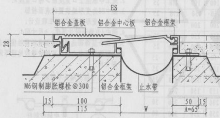
③ 楼、地面 (卡锁式DPC)
